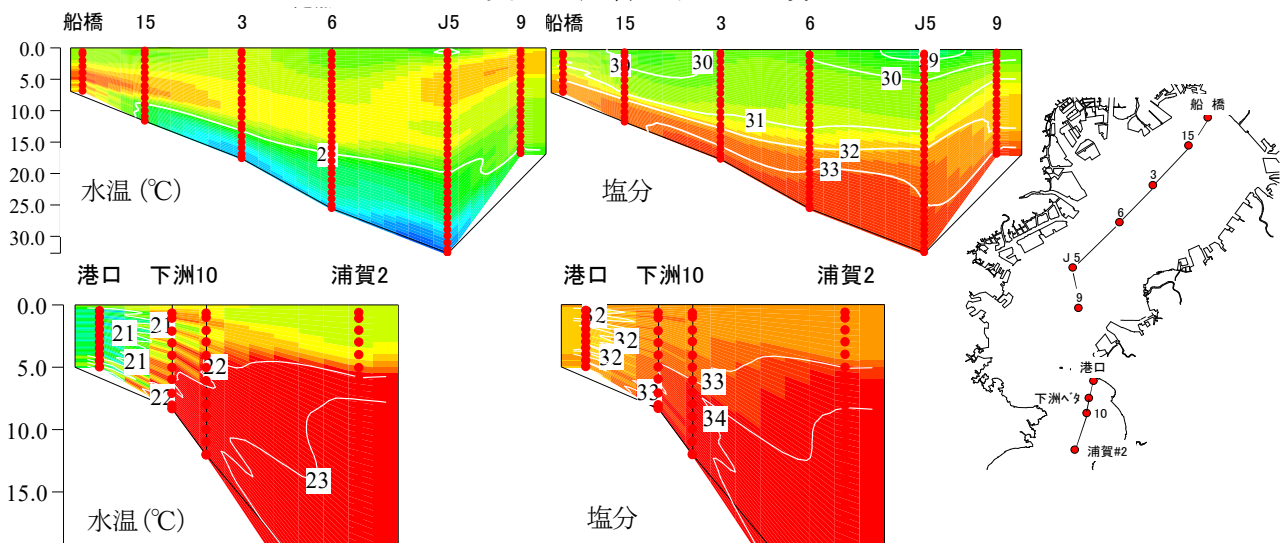
図2 縦断面の水温・塩分
