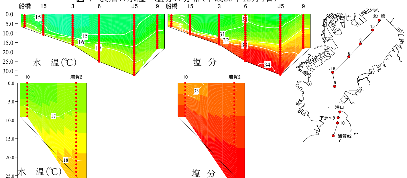
図2 調査ラインの水温・塩分の鉛直分布(平成29年12月4日) (上：内湾、下：内房北部、右：調査ライン)
