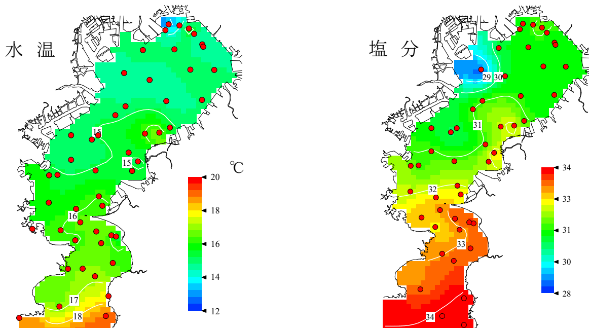
図1 表層の水温・塩分の分布(平成29年12月4日)
