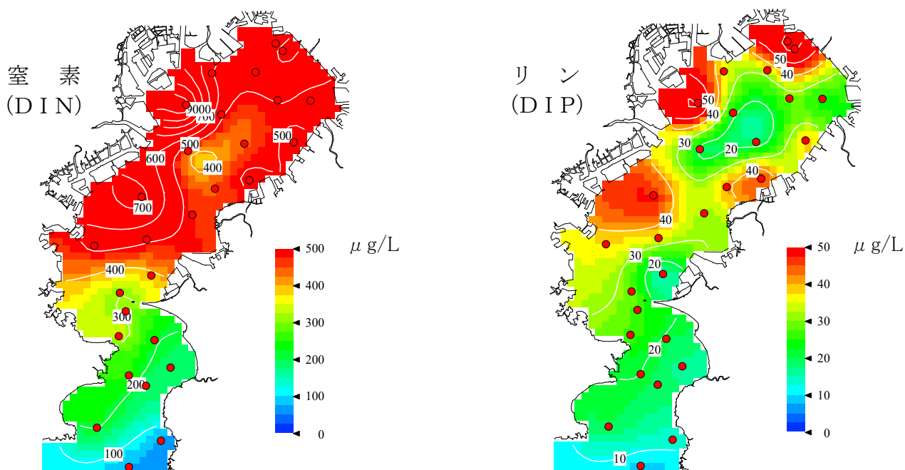
図3 表層の栄養塩濃度の分布(平成29年12月4日)
