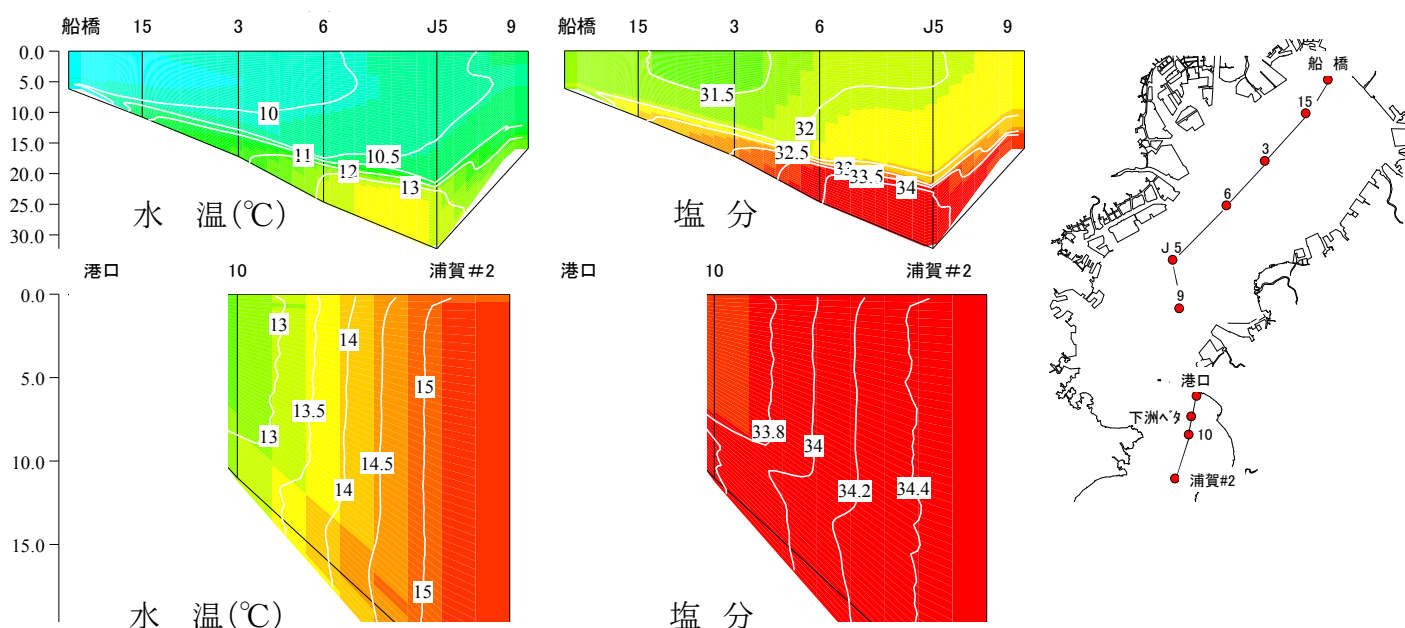
図2 調査ラインの水温・塩分の鉛直分布(平成28年 2月 1- 3日) (上：内湾、下：内房北部、右：調査ライン)
