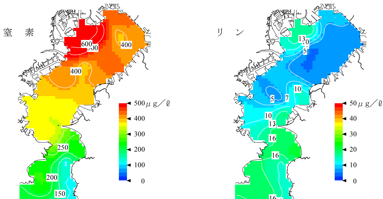
図3 表層の栄養塩濃度の分布(平成28年 2月 1- 3日)
