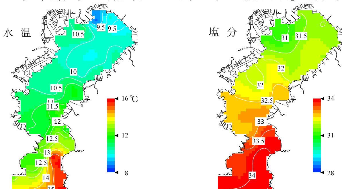
図1 表層の水温・塩分の分布(平成28年 2月 1- 3日)
