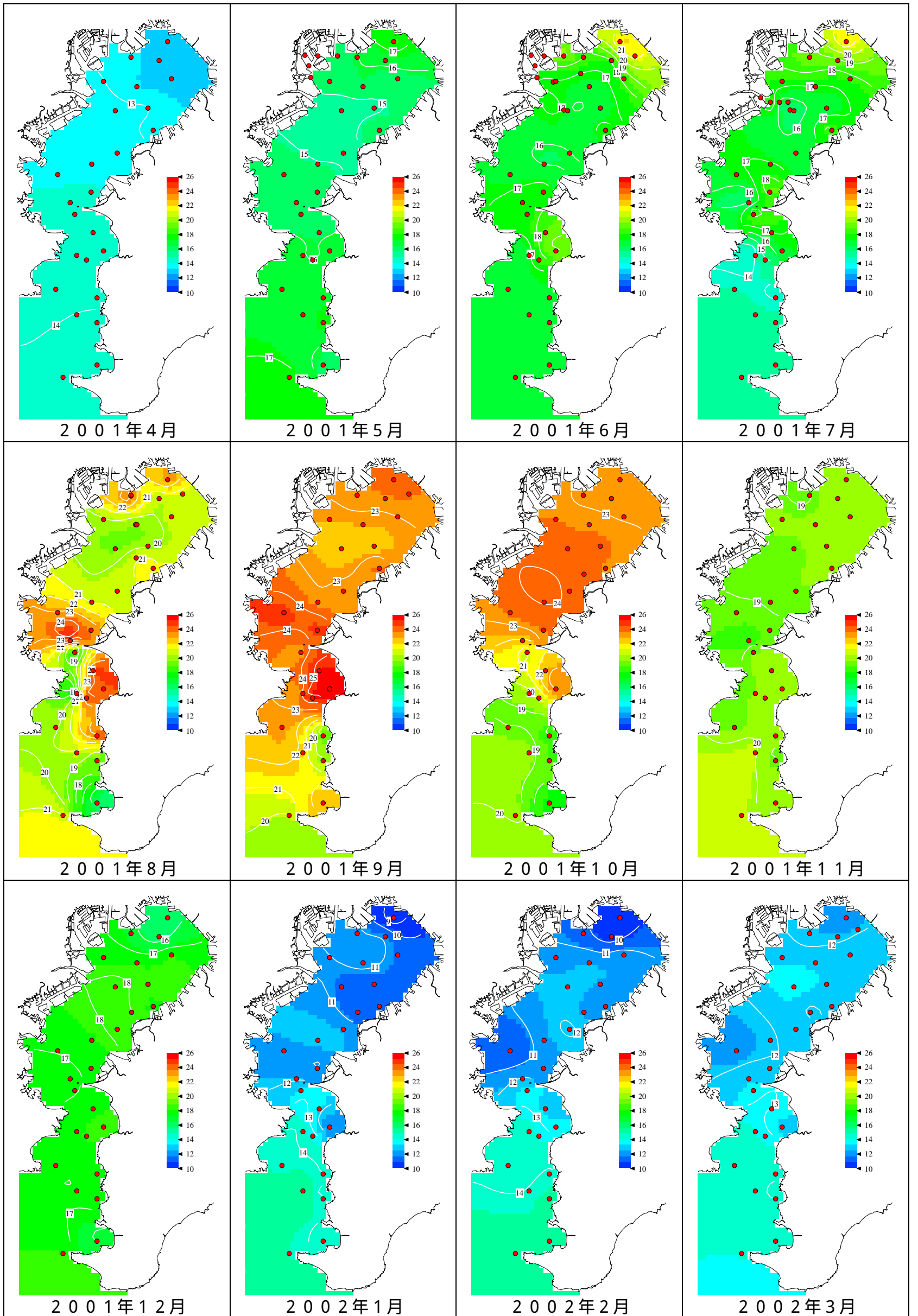
東京湾の水温分布（底層または50m，2001年4月～2002年3月）
