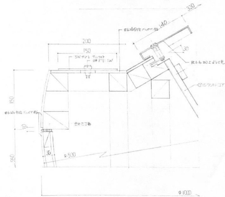
断面詳細図 S-1F
