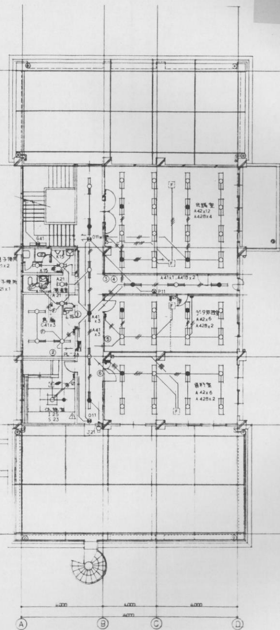
2層平面図 1:100
