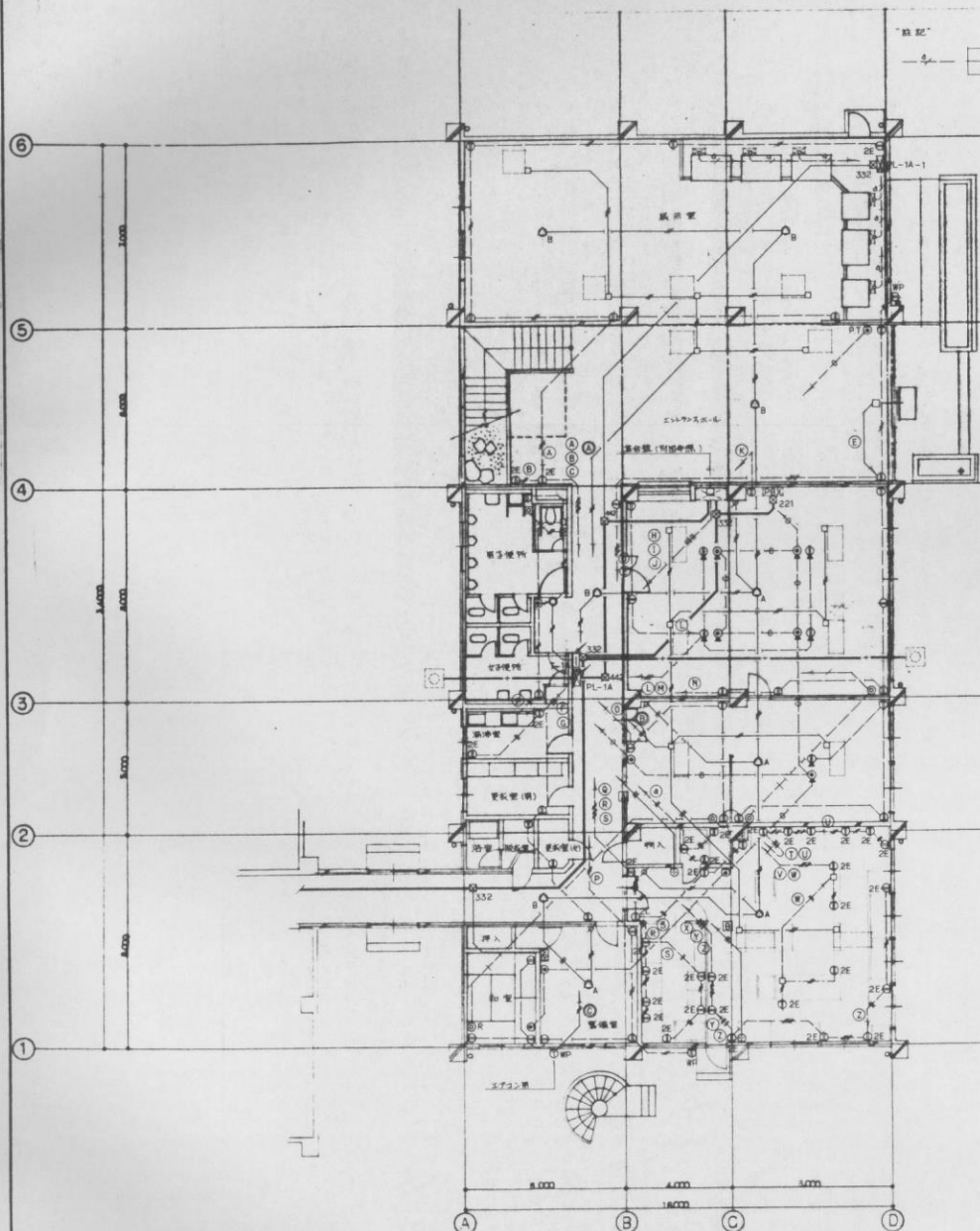
1 階平面図 1:100
