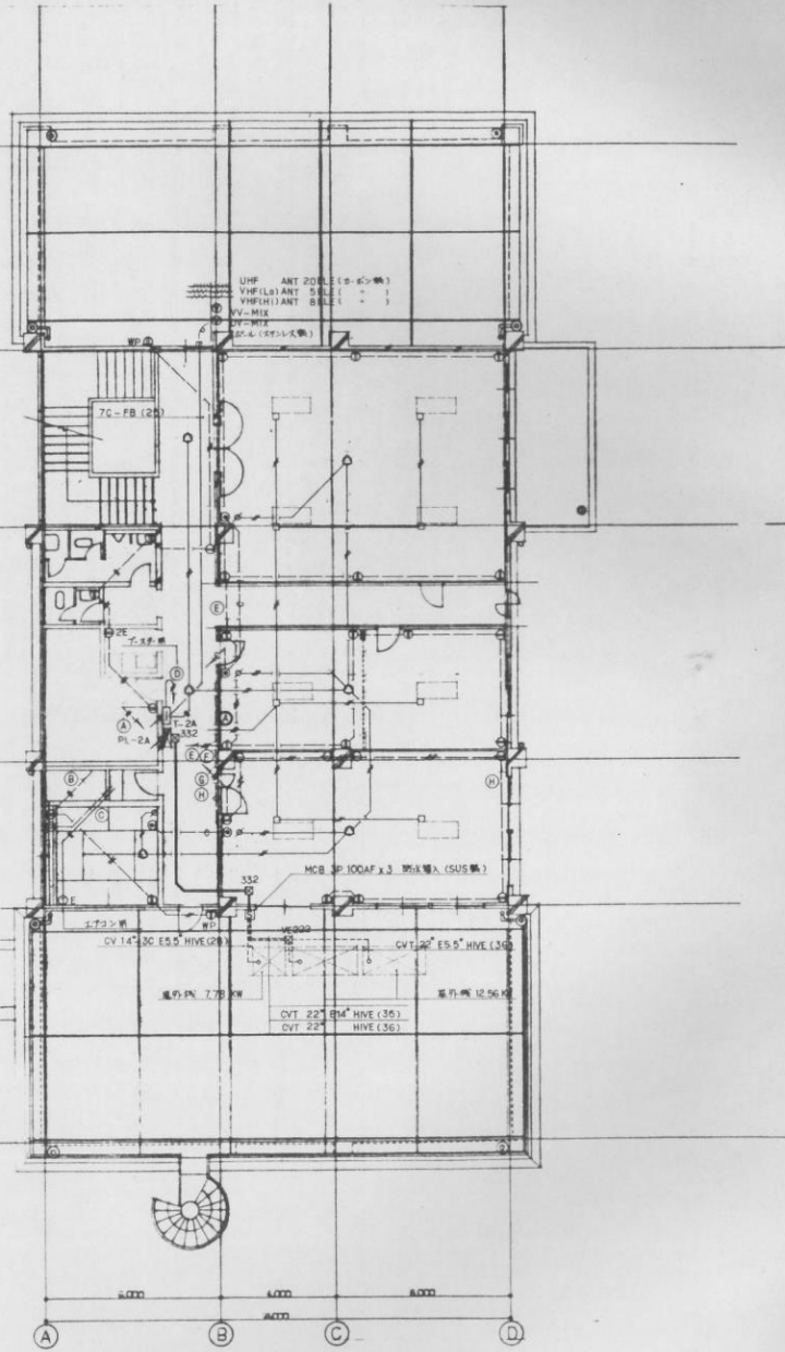
2 階平面図 1:100
