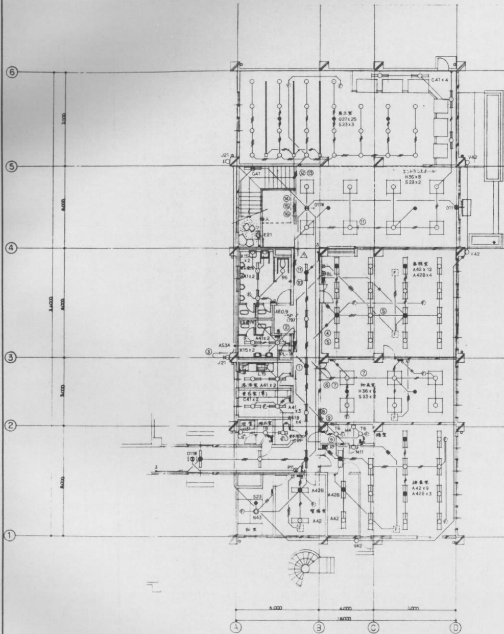
1層平面図 1:100
