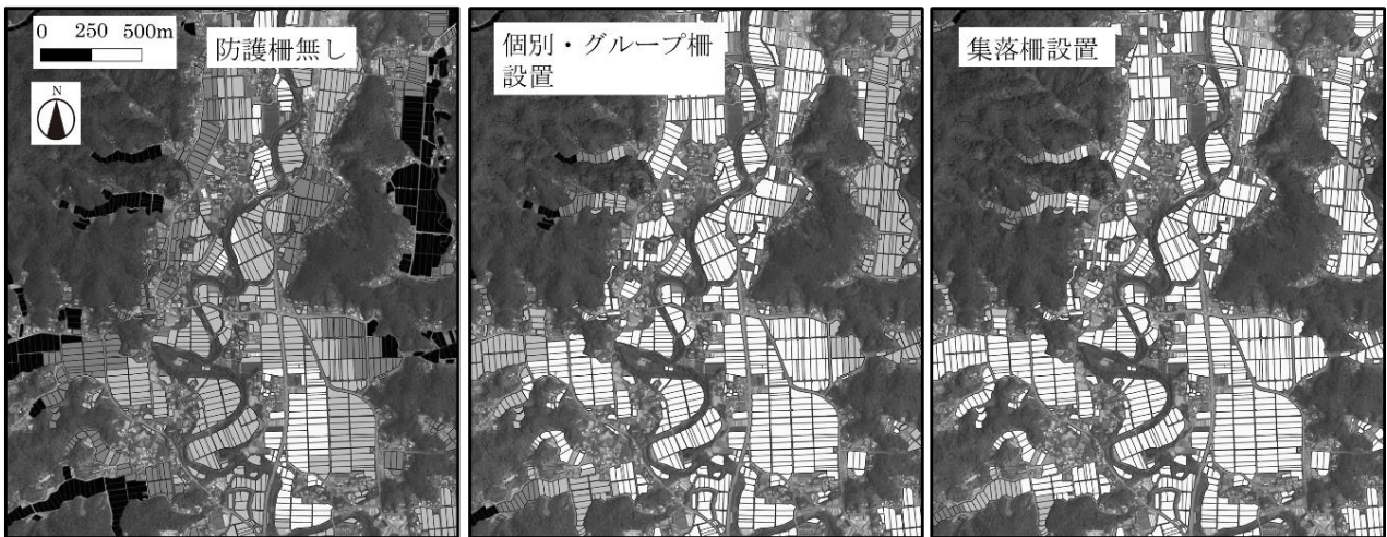
第4図 防護柵無し、個別・グループ柵、集落柵設置を仮定し作成したイノシシ水稲被害発生リスクマップ（一部）
