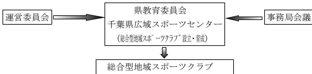
運営組織図
