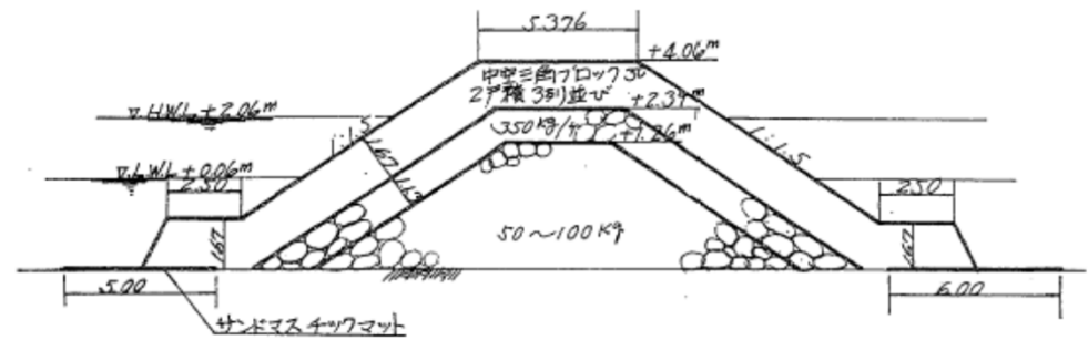
【標準断面図】
