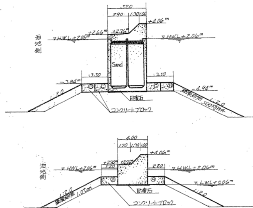
【標準断面図】
