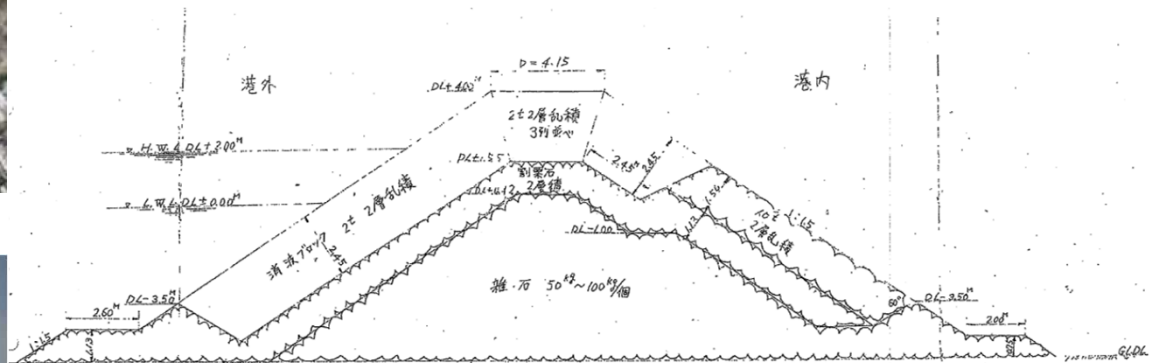
【標準断面図】
