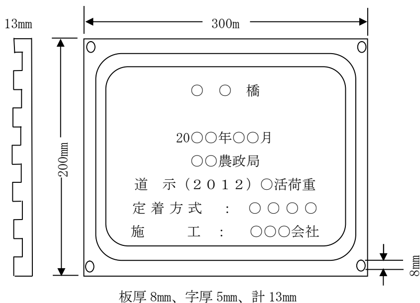
図 12-4-1 橋歴板の記載例
