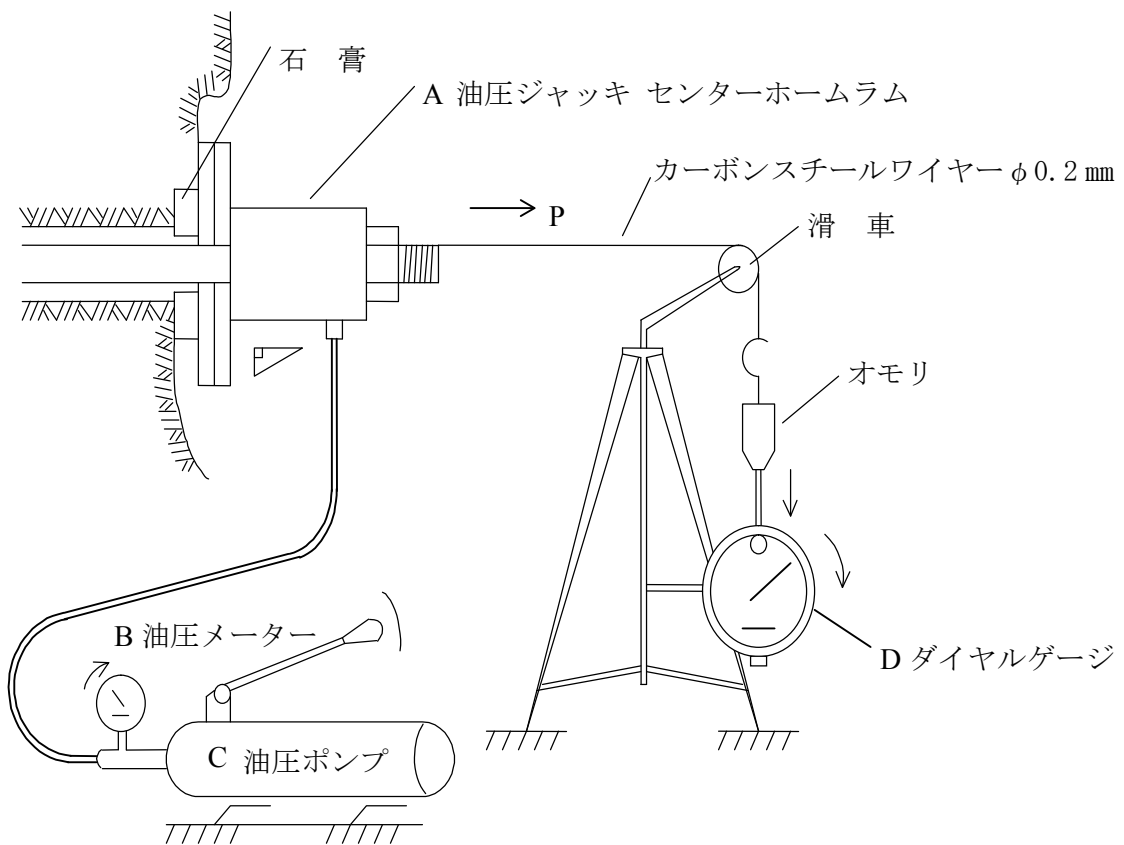
図-29 引抜試験概要図
