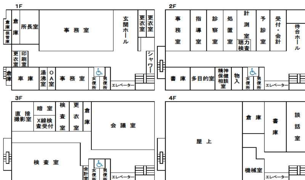
厅舍平面图
