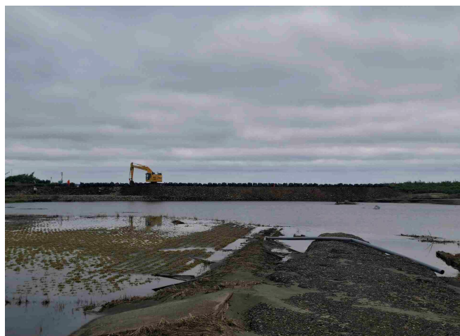
北印旛沼船形干拓における 堤防の荒締切施工状況(2)
