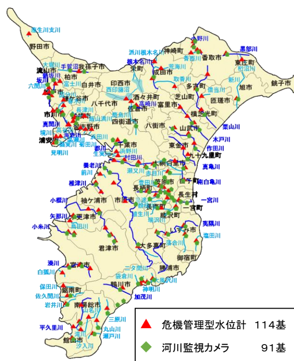
危機管理型水位計・河川監視カメラ設置箇所図
