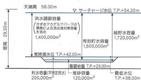
＊矢那川ダム貯水池容量配分
