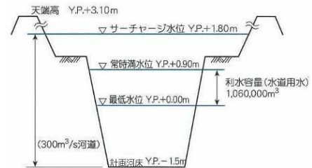
＊黒部川貯水池断面図
