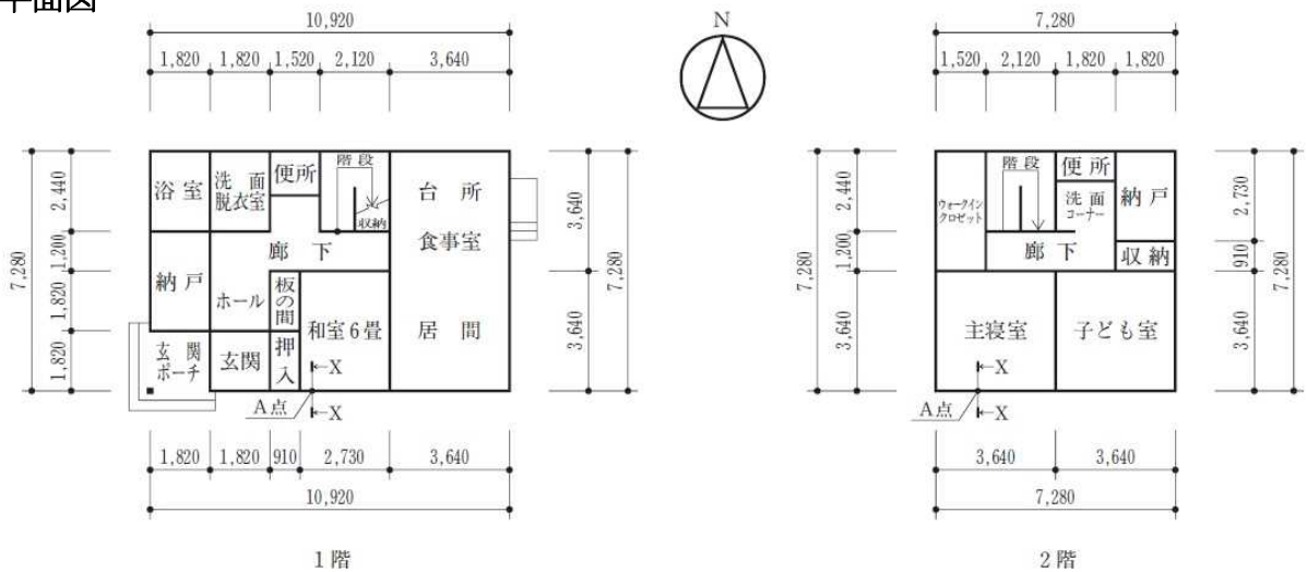
各階平面図
