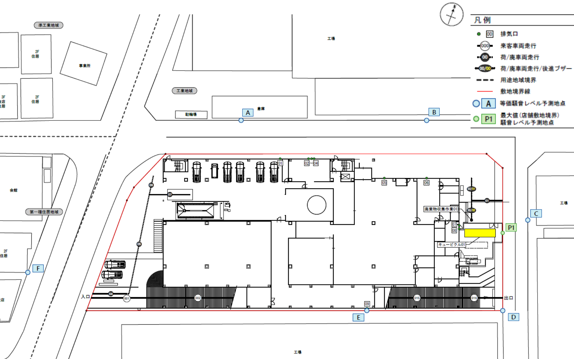
図5-1 騒音発生源及び予測地点位置図(1階)
