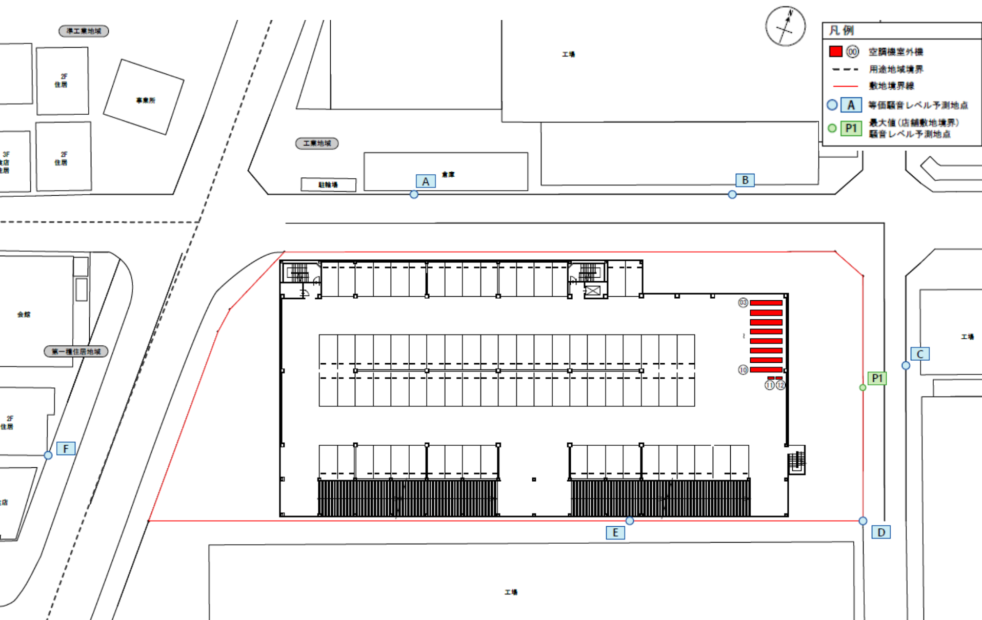
図5-3 騒音発生源及び予測地点位置図(4階)
