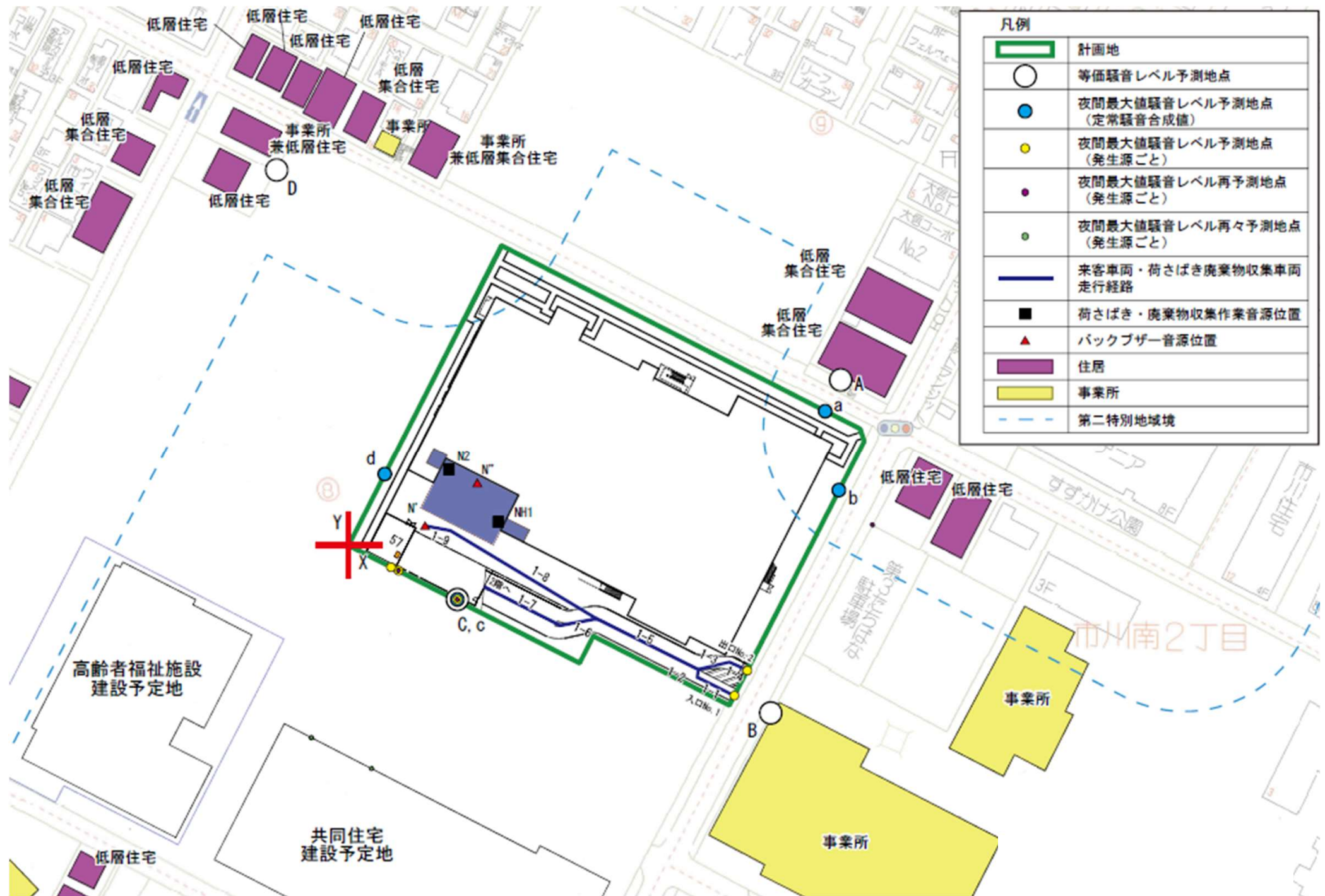
図5-1 騒音発生源及び予測地点位置図(1階)
