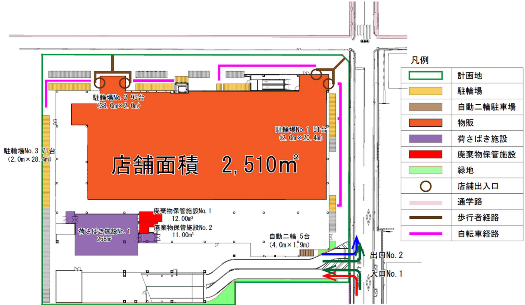
図3—1 建物配置図・平面図(1階)
