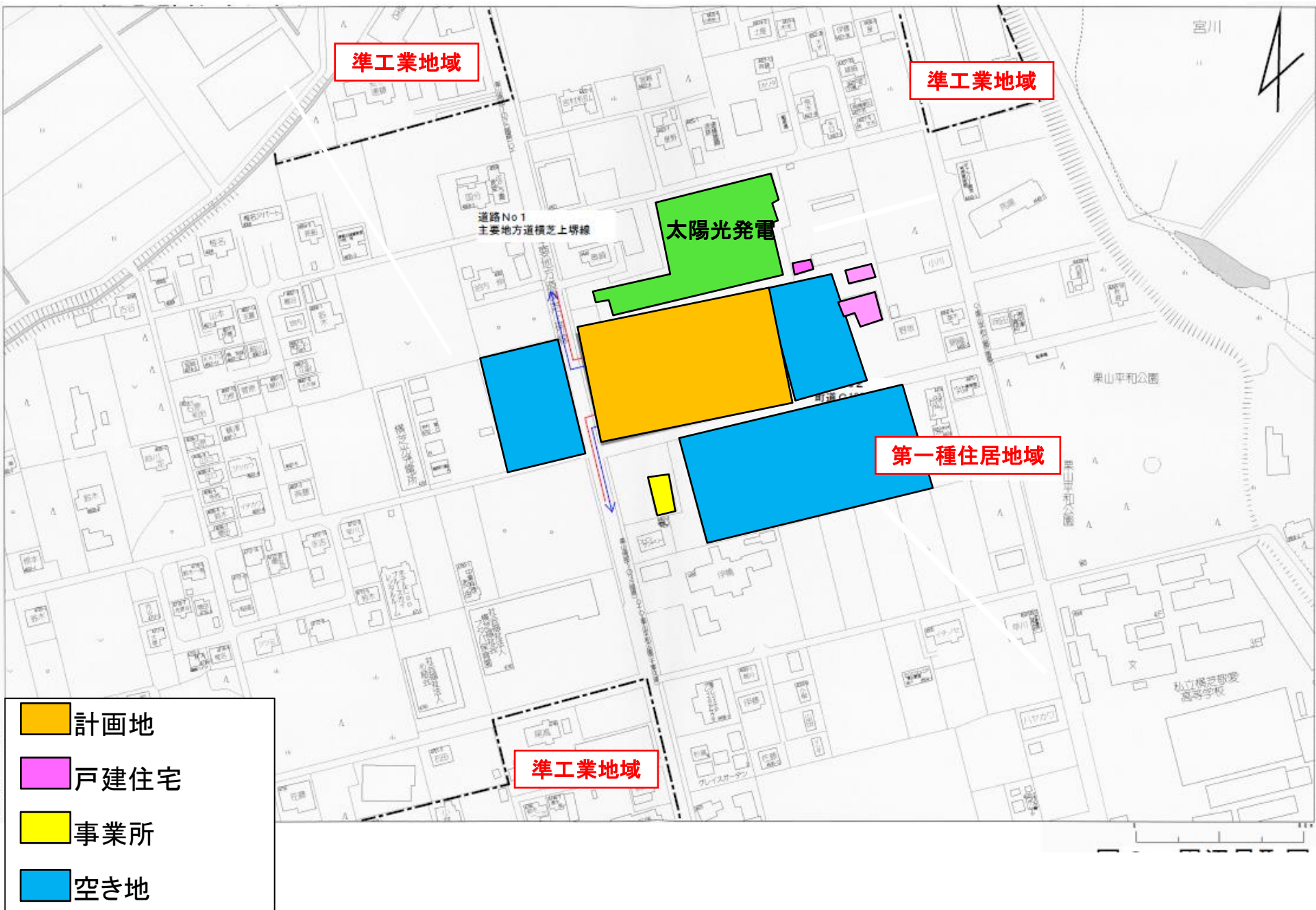
図2 周辺見取図
