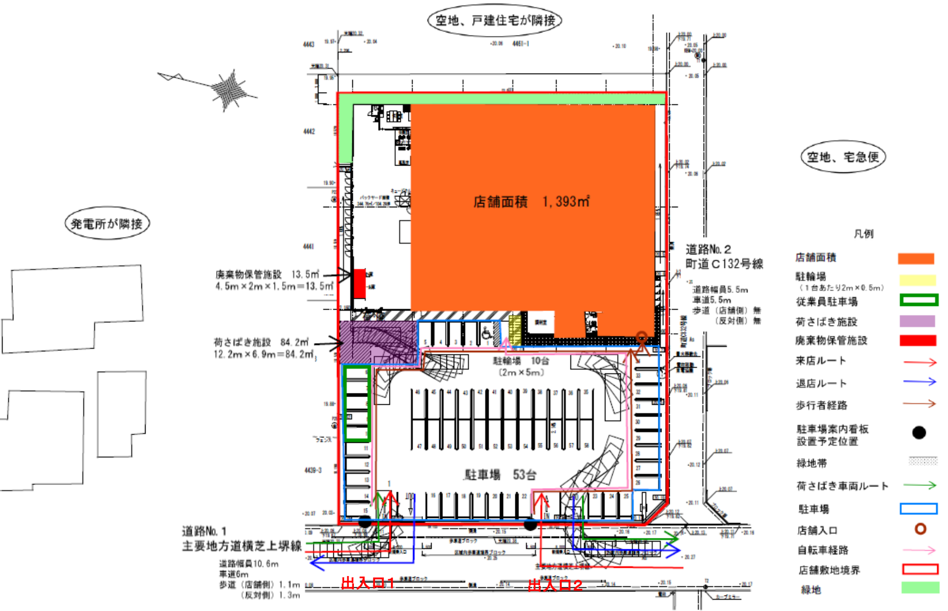
図3 建物配置図
