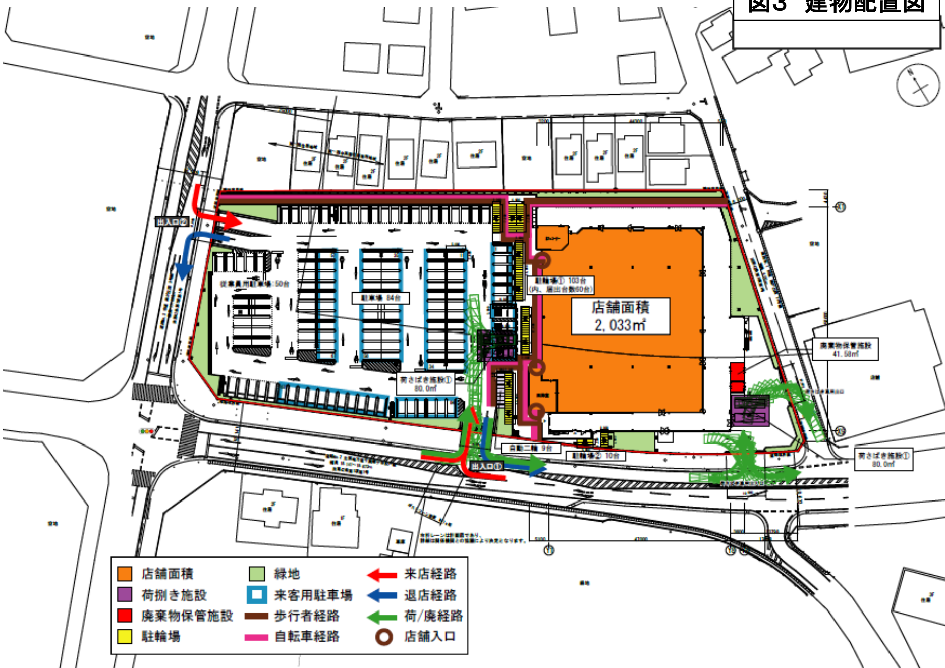
図3 建物配置図
