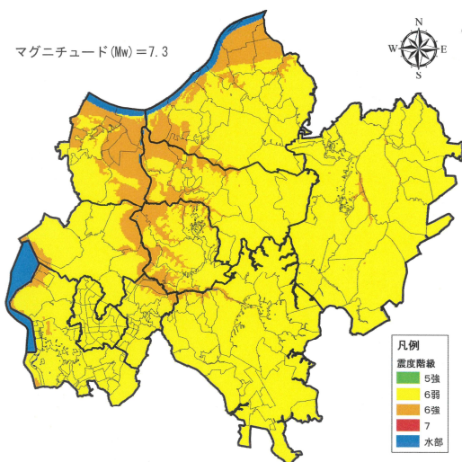
【成田空港直下地震 震度段階図】
