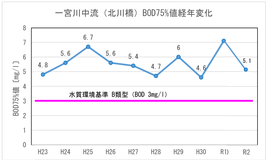
■ 環境基準が未達成の中流での水質経年変化
