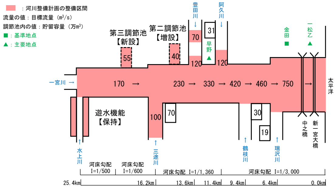
■ 河川整備計画における目標流量配分図
