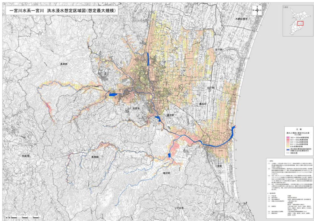
■ 一宮川浸水想定区域図（令和元年12月23日公表）
