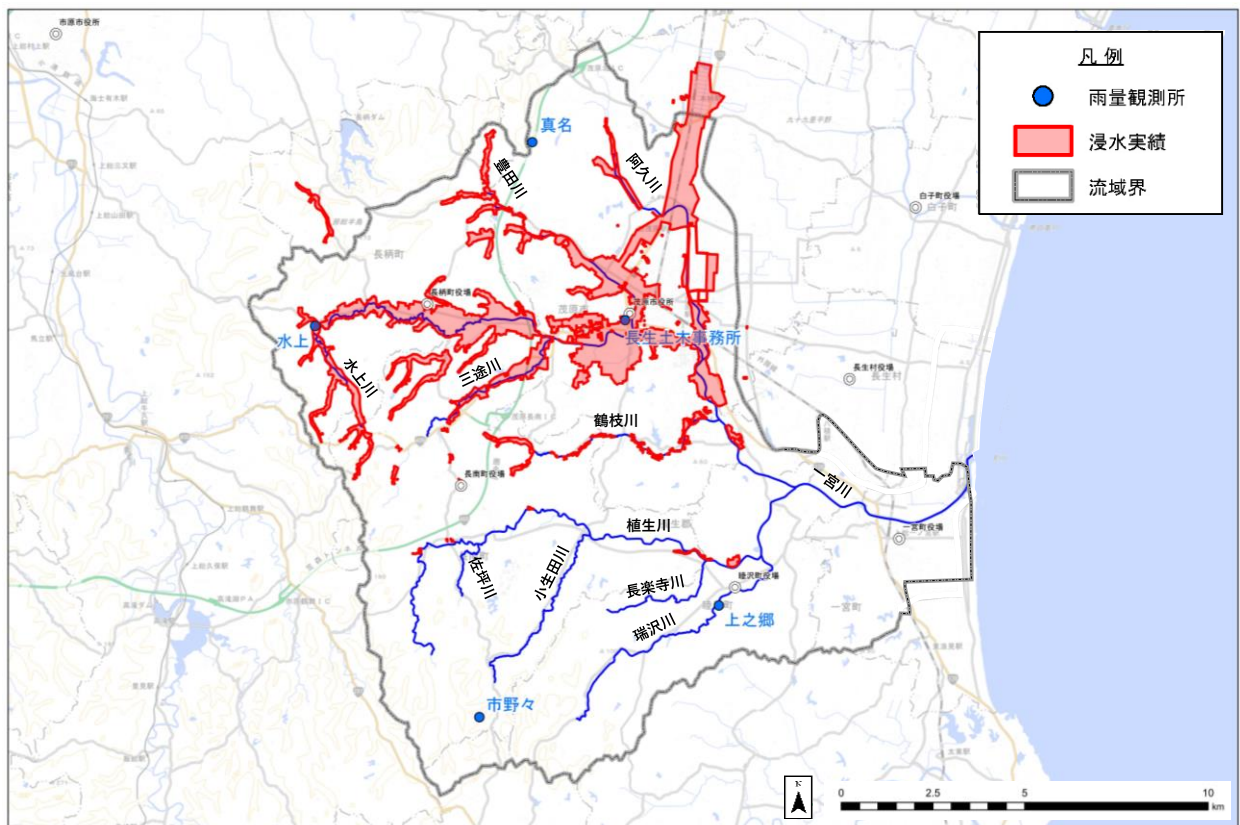
■令和元年10月豪雨の浸水区域
