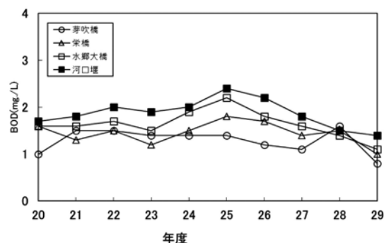
図表 4-3-11 利根川の主要地点の水質経年変化 (BOD年平均値)
