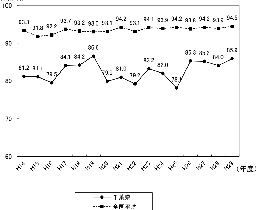
図表 4-4-18 地下水の環境基準達成率
