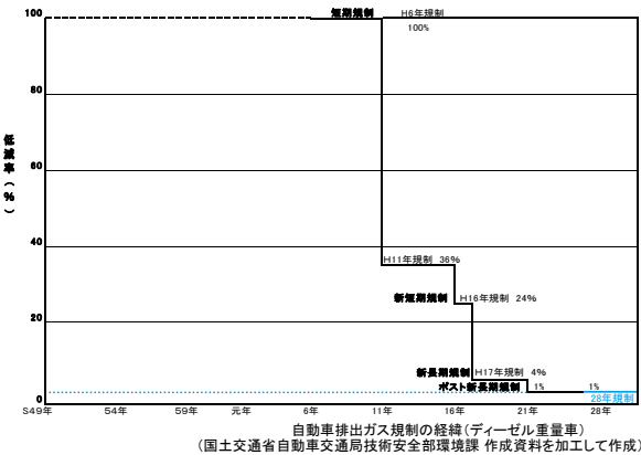
図表 4-1-34 PM排出ガス規制の強化
