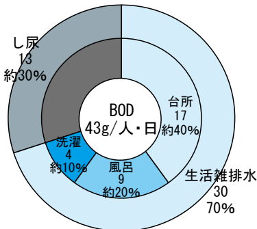
図表 4-3-20 生活排水の性状
