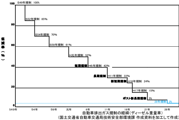
図表 4-1-33 NO x 排出ガス規制の強化
