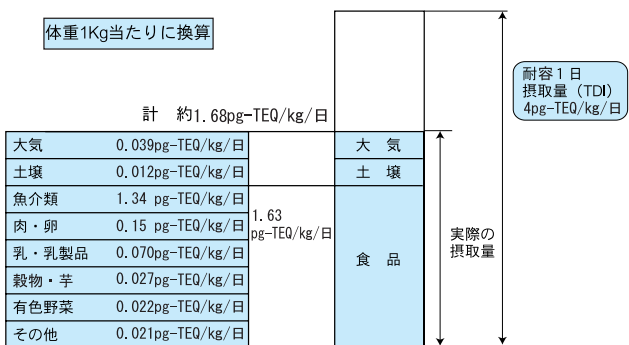
図2-12-5 我が国におけるダイオキシン類の1人1日摂取量
