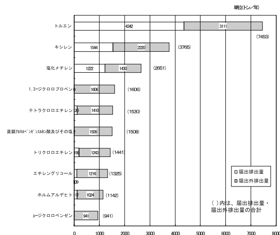
図2-12-2 届出排出量・届出外排出量上位10物質とその量
