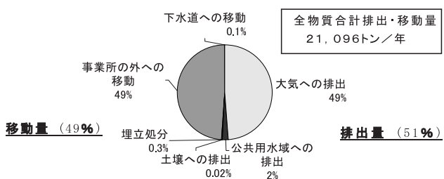
図2-12-1 届出排出量・移動量の排出先・移動先別内訳（平成13年度排出分）
