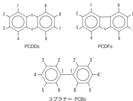
図2-12-4 ダイオキシン類の構造図
