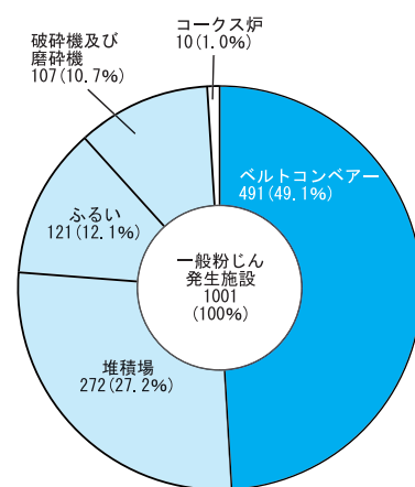
図2-5-2 一般粉じん発生施設の種類別状況 (千葉市・船橋市を除く16年3月末現在)
