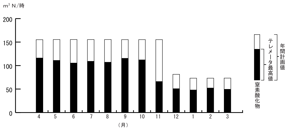
図2-5-19 年間計画値とテレメータ最高値（覚書締結4工場合計）の月別推移（15年度）
