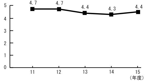
図2-5-14 降下ばいじん量の年平均値の年度別推移
