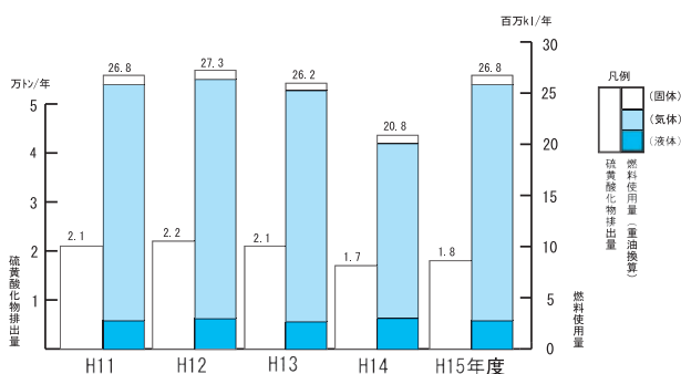
図2-5-3 県内主要工場・事業場における硫黄酸化物排出量及び燃料使用量の経年変化
