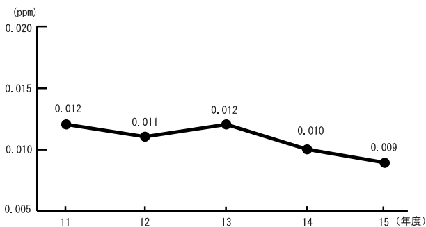
図2-5-6 一酸化窒素の年平均値の年度別推移（一般環境大気測定局）
