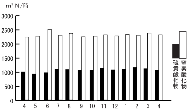
図2-5-17 月別排出量の推移
