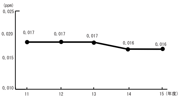
図2-5-4 二酸化窒素の年平均値の年度別推移（一般環境大気測定局）
