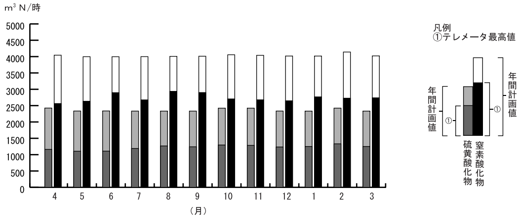
図2-5-19 年間計画値とテレメータ最高値（覚書締結4工場合計）の月別推移（15年度）
