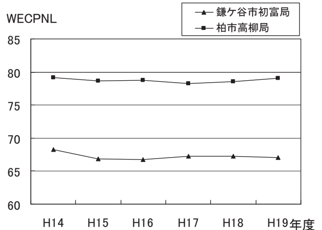
図表 4-2-15 下総飛行場周辺航空機騒音測定結果の推移
