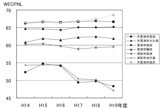
図表 4-2-14 羽田空港周辺航空機騒音測定結果の推移
