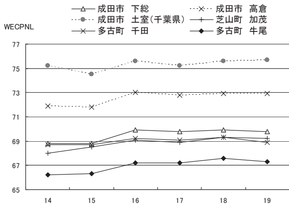
図表 4-2-13 暫定平行滑走路側年間WECPNL値の推移
