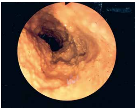
尿石で覆われて狭くなった排水管内部
