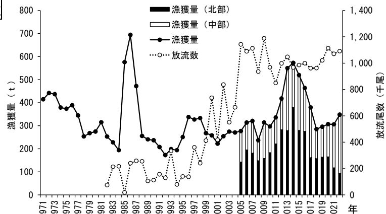
千葉県におけるヒラメ漁獲量と放流尾数の経年変化
