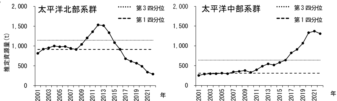
太平洋北部系群及び太平洋中部系群における推定資源量の経年変化
