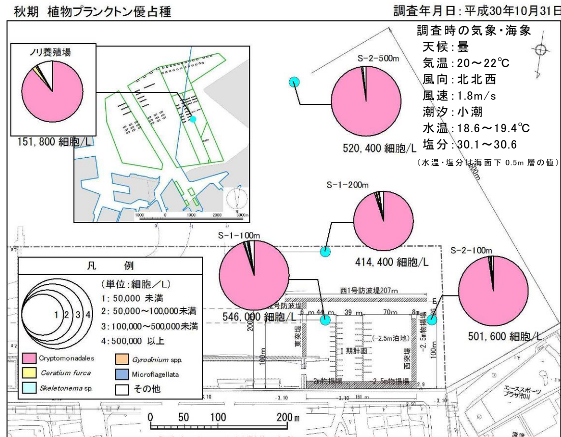
図3 植物プランクトンの優占種の出現状況
