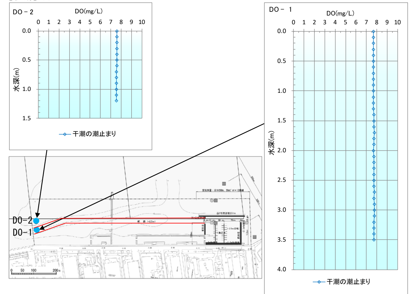
図 4 溶存酸素量 (DO) の鉛直観測結果
