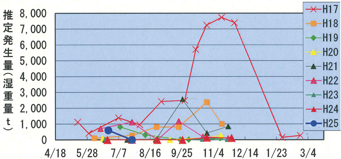
図1 三番瀬調査域内のアオサ推定発生量(湿重量, t)の推移
