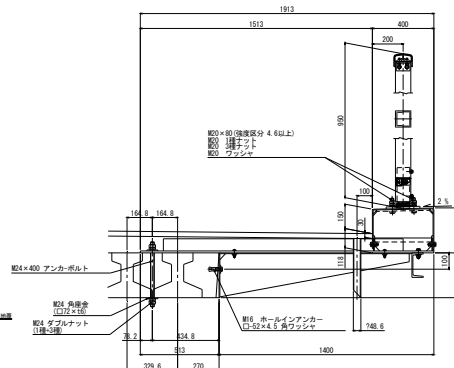
標準設置断面図
