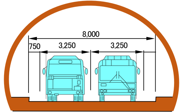
新実入トンネル横断面図
