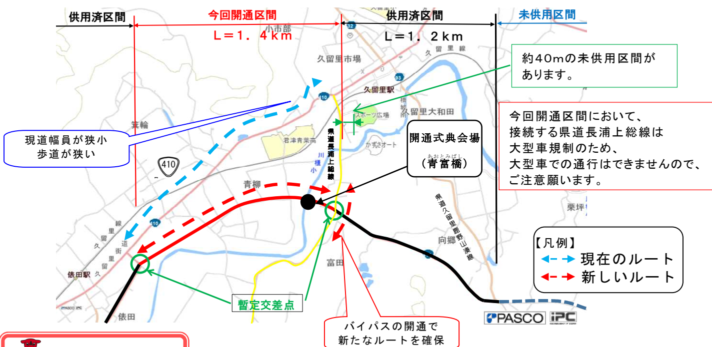
国道410号久留里馬來田バイパス
