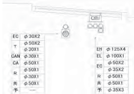
標準断面図
