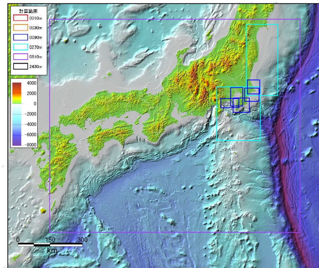
図 8-1 内閣府（2013）による津波の計算範囲（90m～2430m メッシュ領域）
