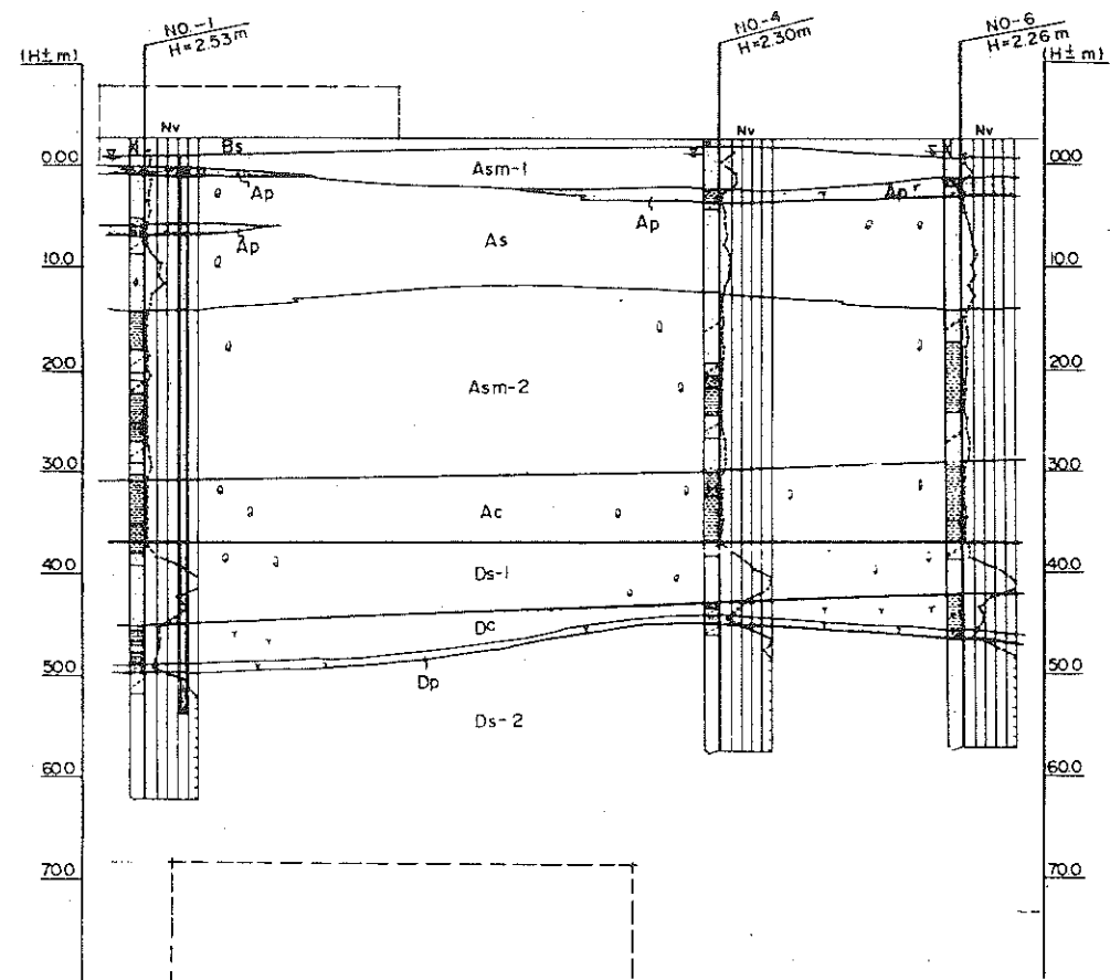
C-C'断面
