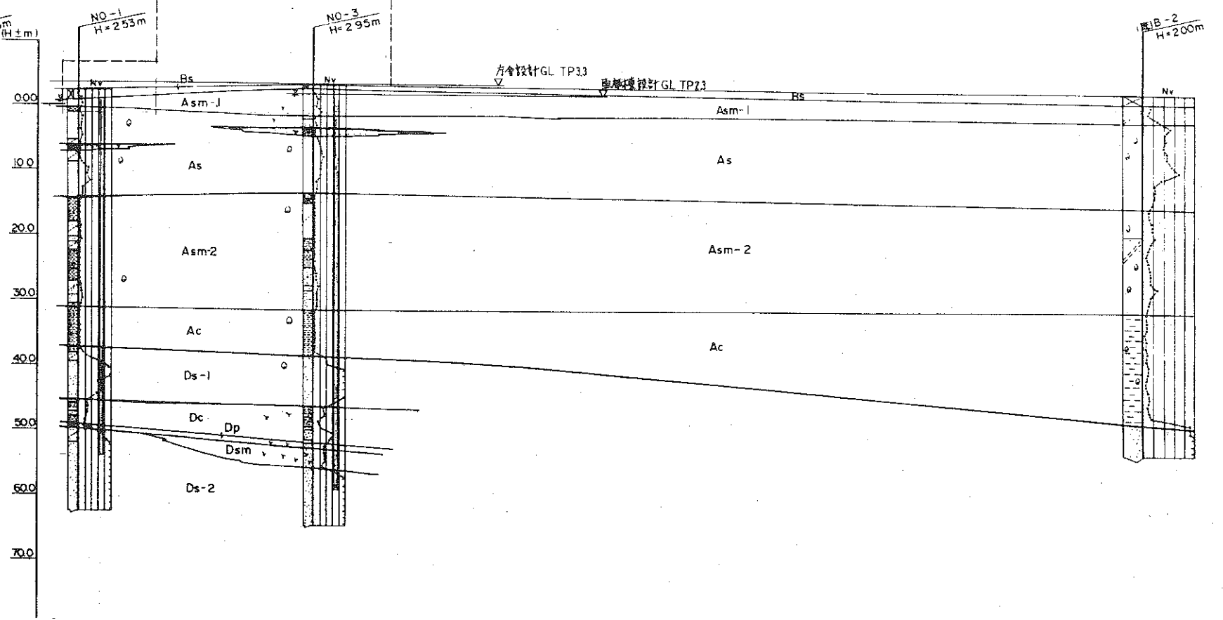
D-D'断面
