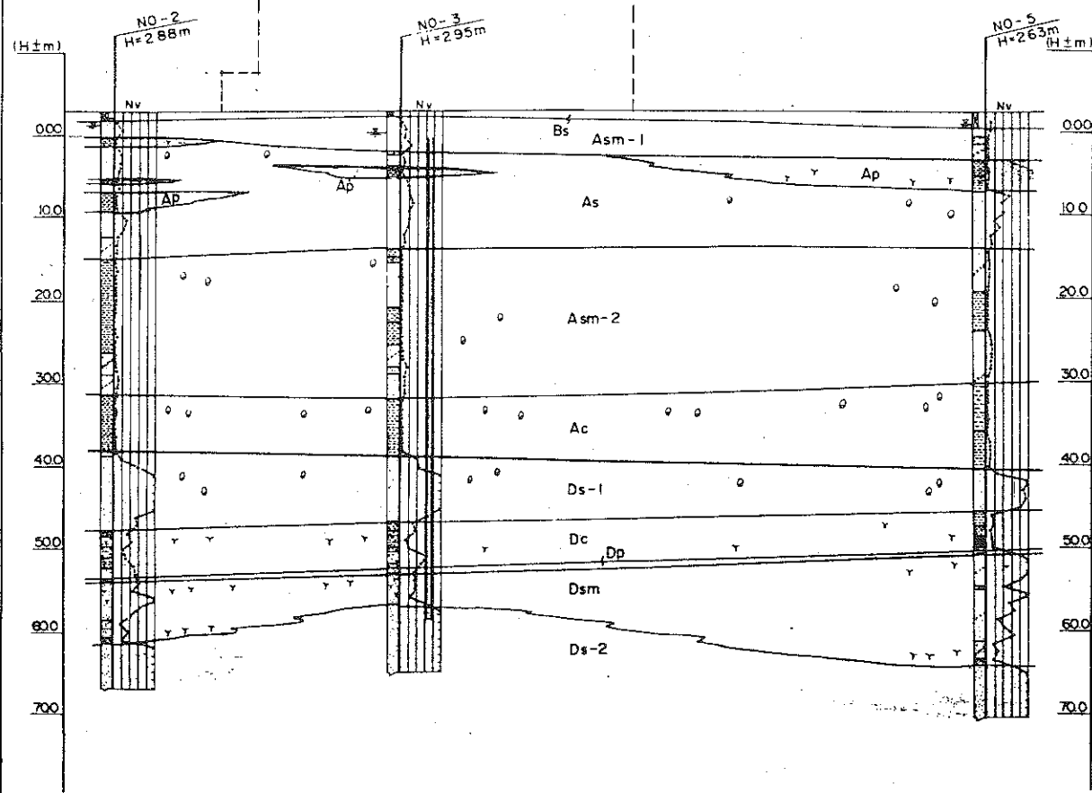
C-C'断面
