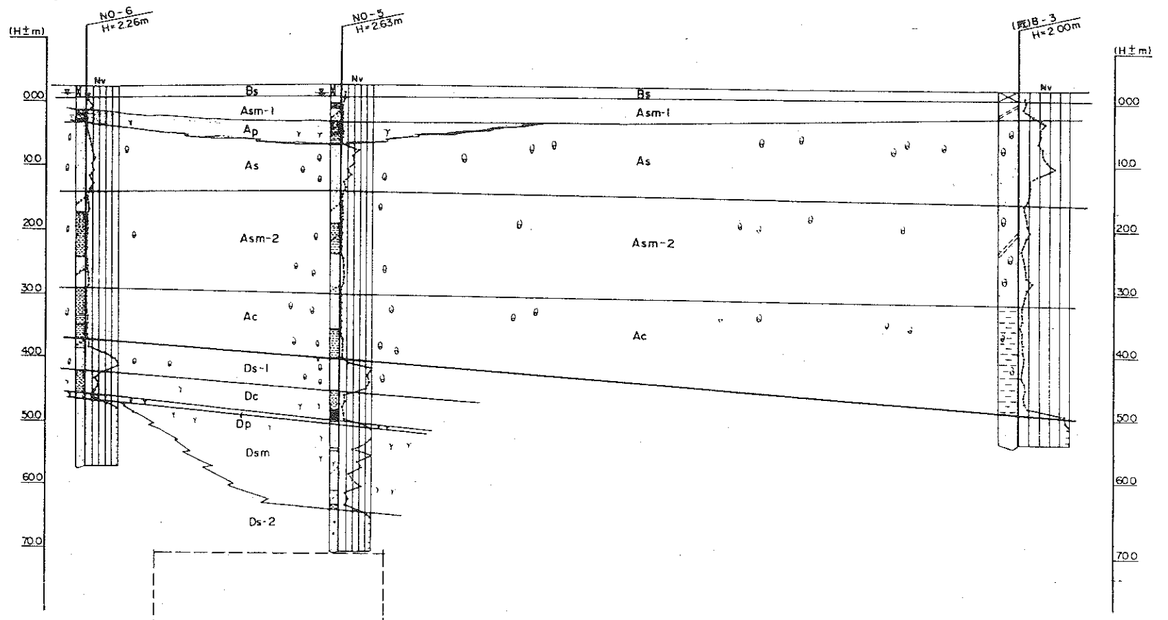
B-B'断面
