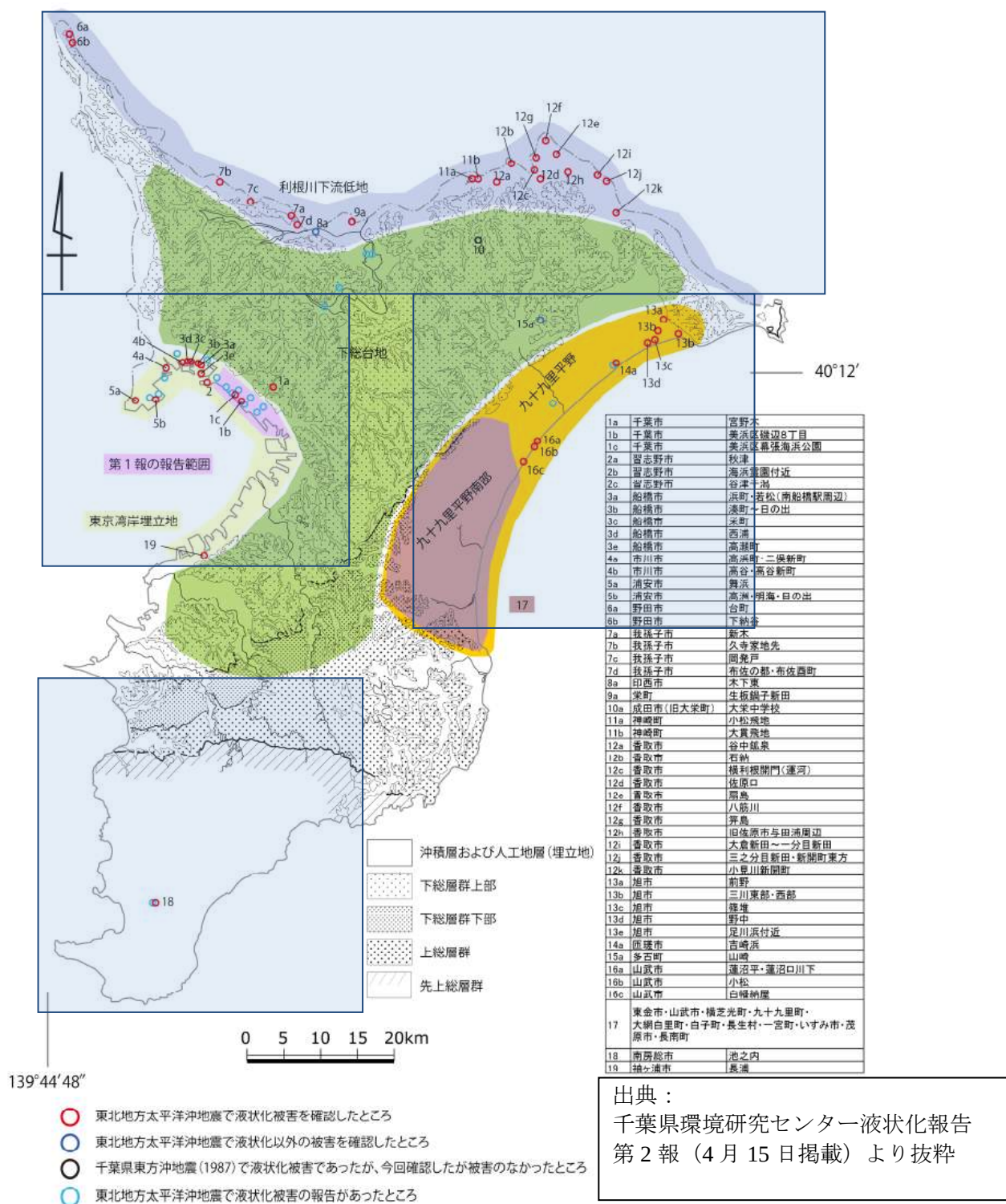
図-2.4.3 千葉県内における液状化-流動化被害分布とその地域区分及び調査位置
