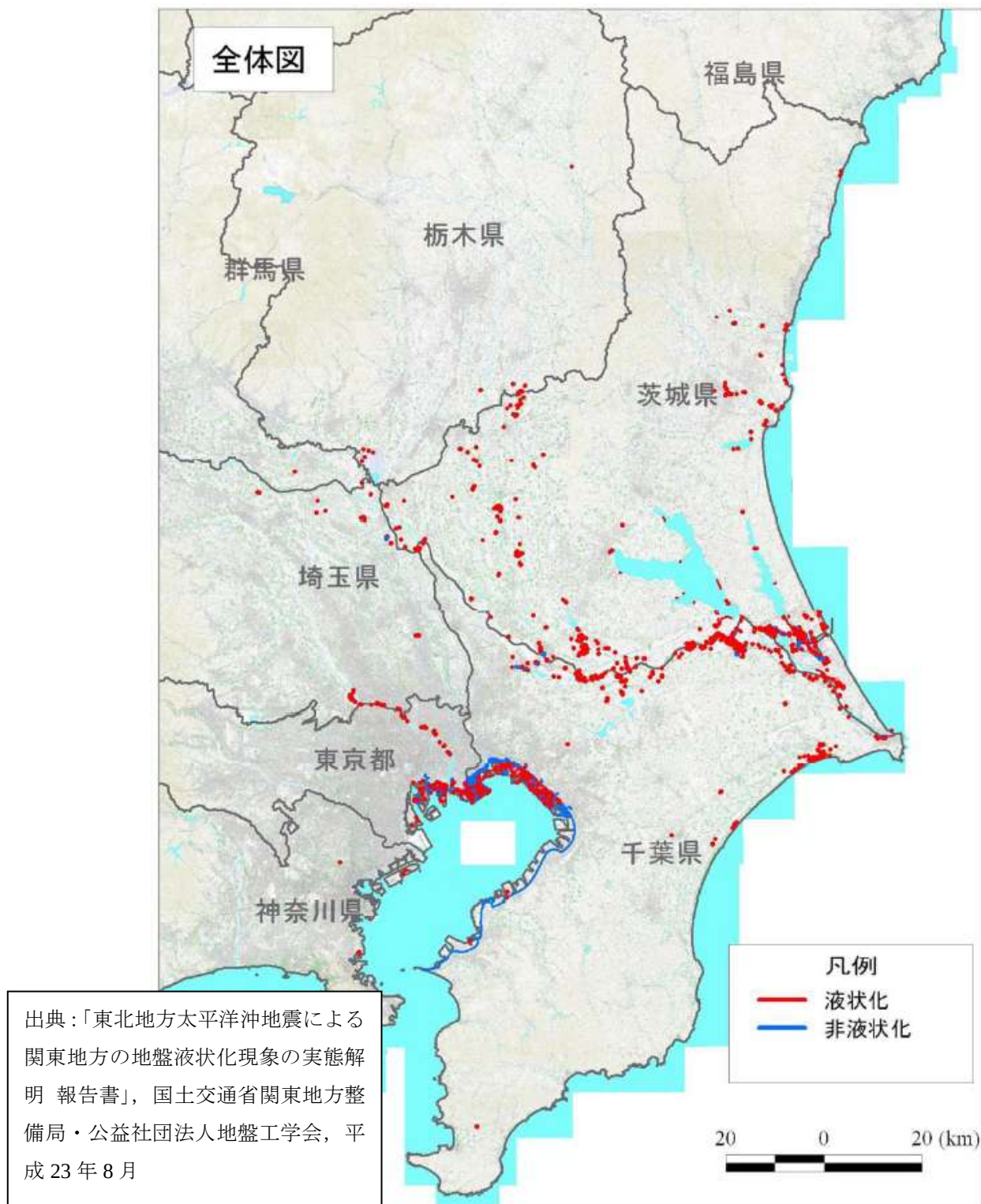
図 2.1 関東地方で液状化現象が認められた地点，及び地域
