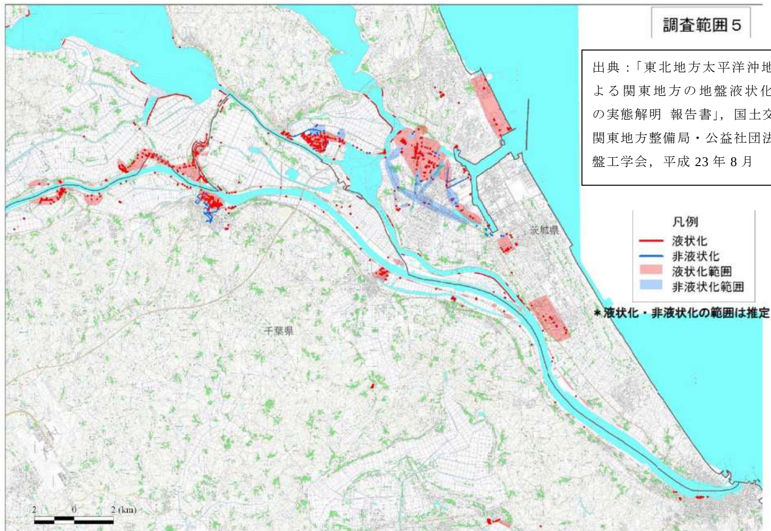
図 2.3.5 液状化調査範囲位置図その 5（利根川下流域（佐倉～銚子），霞ヶ浦南東部）
