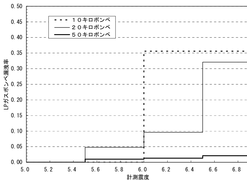
図 11.5-2 LP ガスボンベ漏洩率関数
