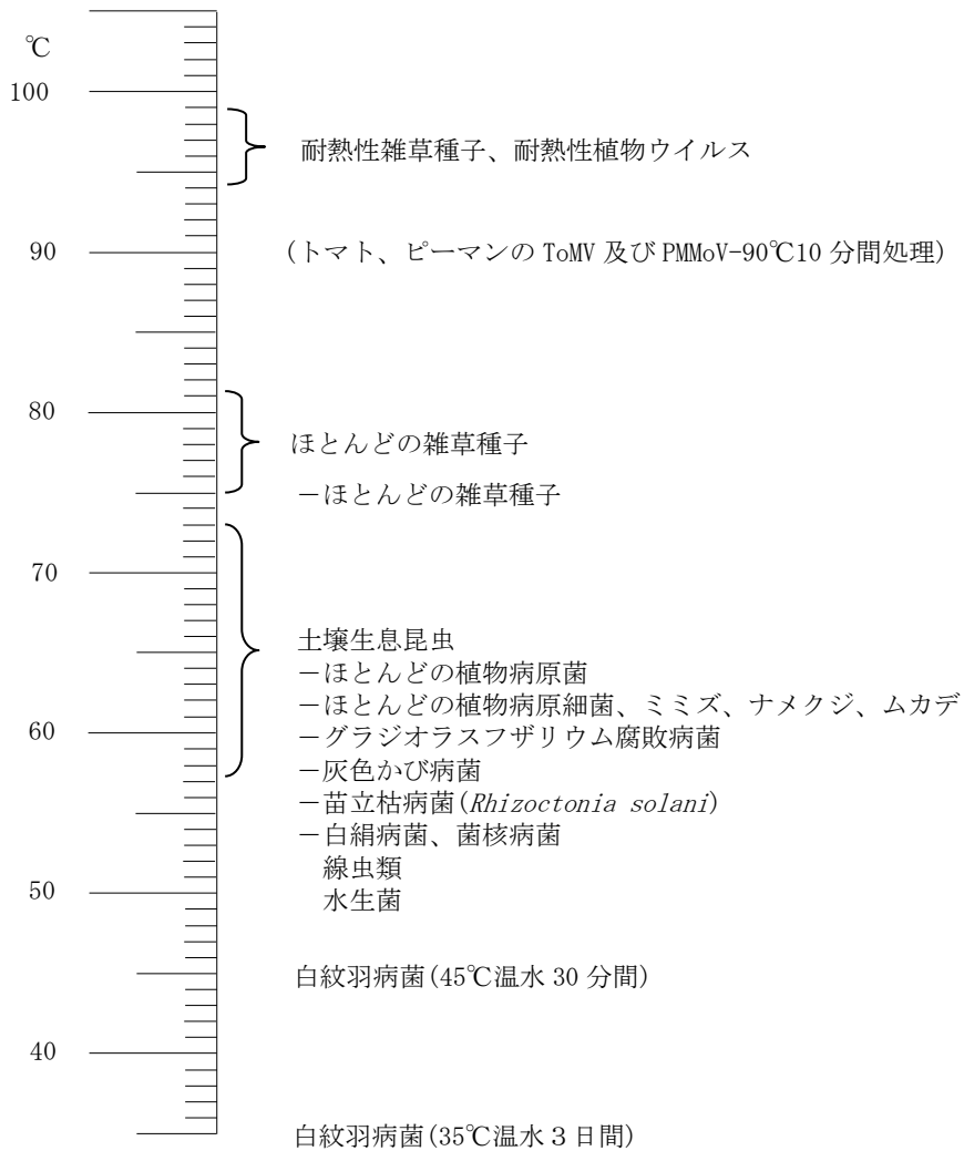
図 有害動植物の死滅温度(湿熱 30分間)
