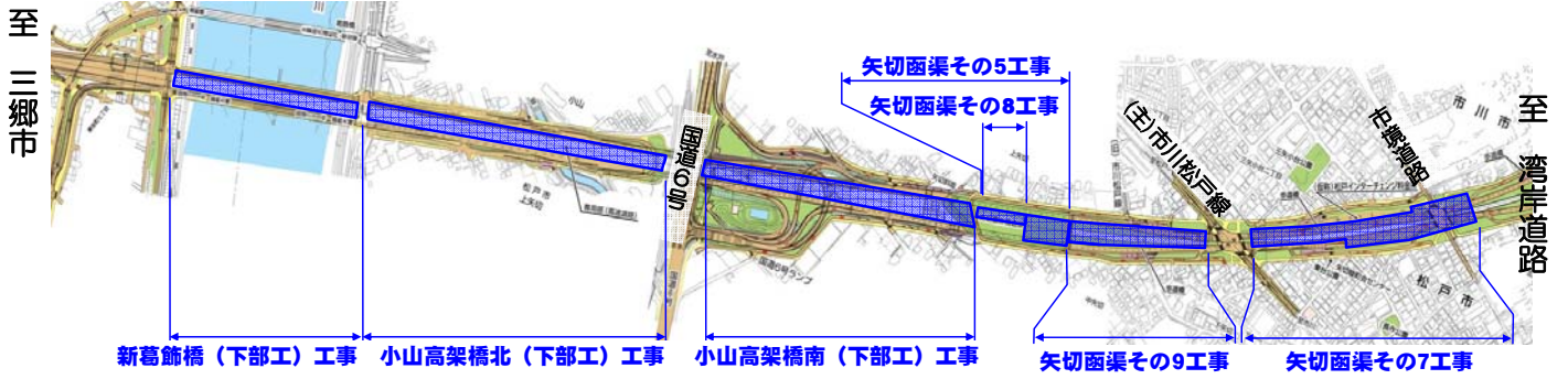
小山高架橋南（下部工）工事の工事範囲 小山高架橋北（下部工）工事の工事範囲
