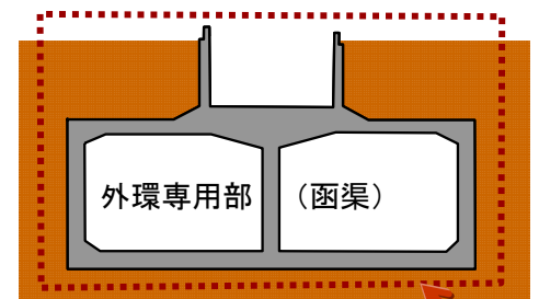
堀之内地区函渠その4工事の工事範囲
