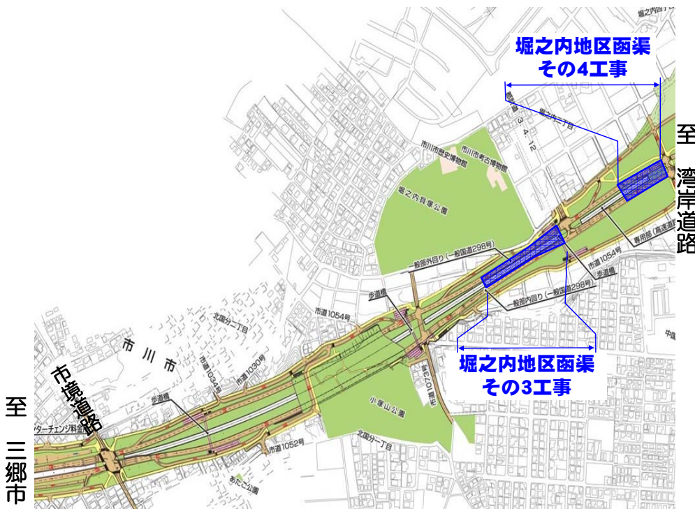
堀之内地区函渠その3工事の工事範囲
