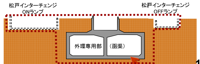
矢切函渠その7工事の工事範囲
