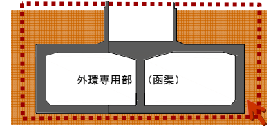
矢切函渠その9工事の工事範囲
