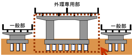
小山高架橋南（下部工）工事の工事範囲 小山高架橋北（下部工）工事の工事範囲
