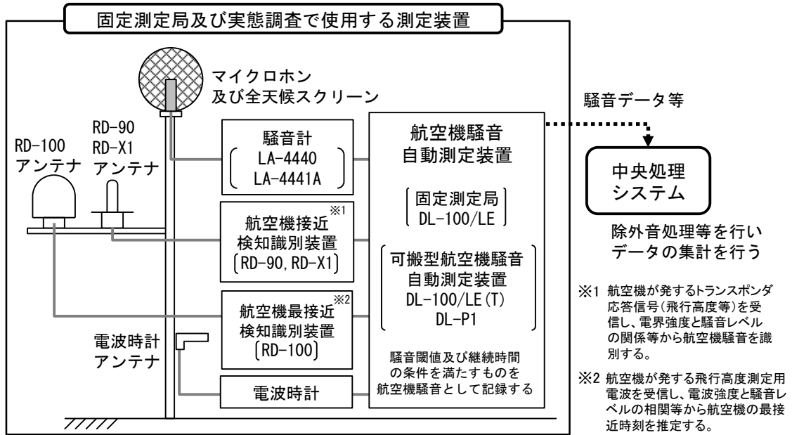
図2 基本構成図
