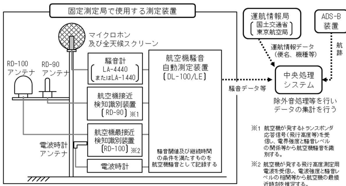
図2 基本構成図
