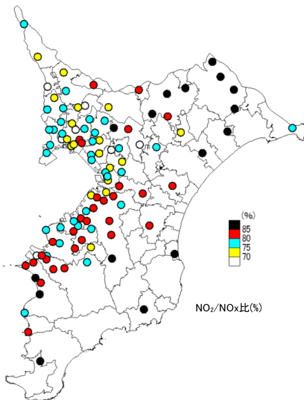
図2-2-10 NO 2 /NO x 比の分布(一般局)
