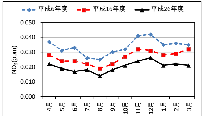
図2-2-4 NO 2 月平均値の経月変化(自排局)
