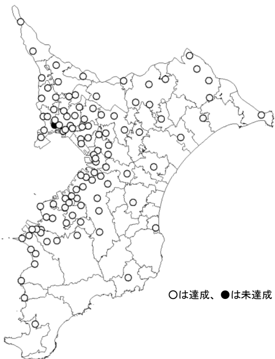
図2-2-7 環境目標値達成の状況(一般局)
