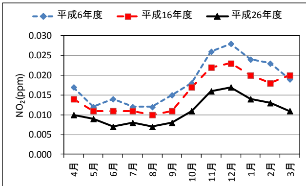
図2-2-3 NO 2 月平均値の経月変化(一般局)
