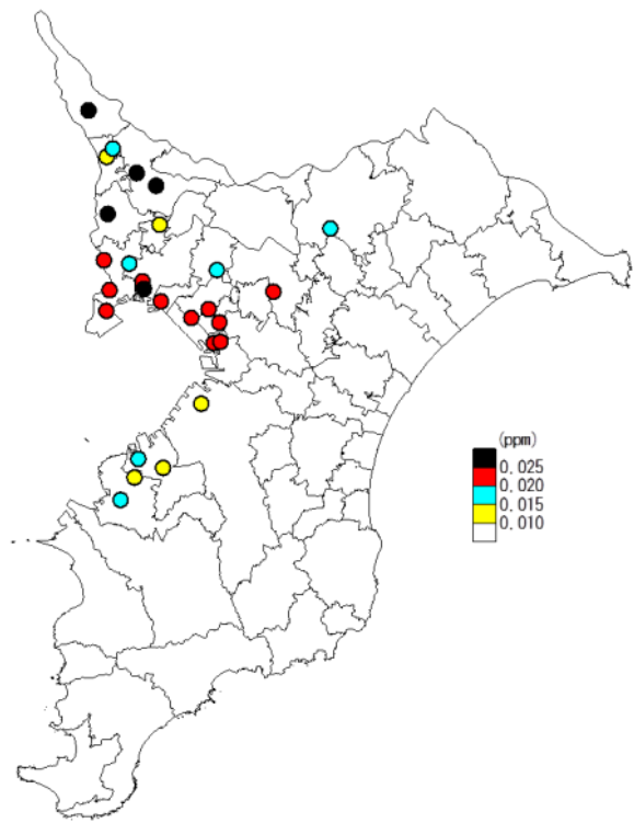
図2-2-2 NO 2 年平均値の分布(自排局)
