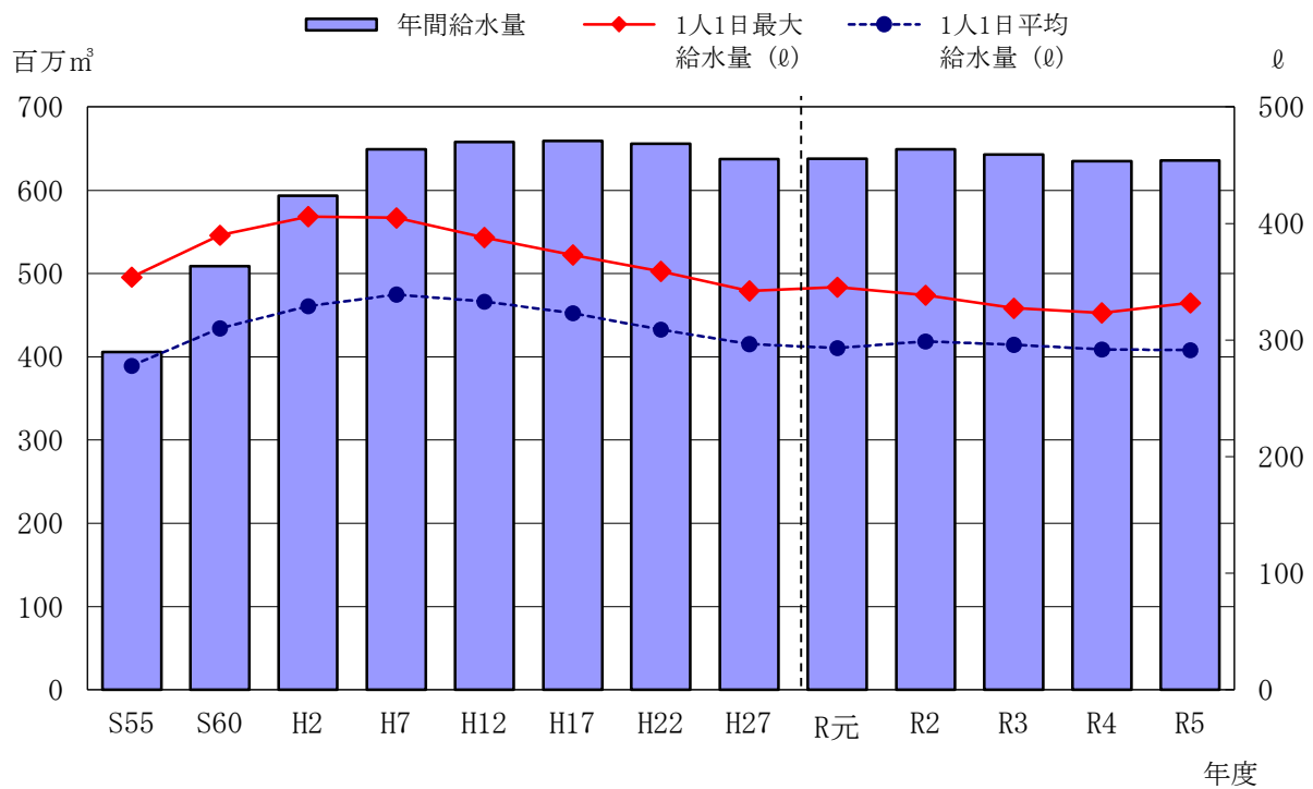
図-5 給水量
