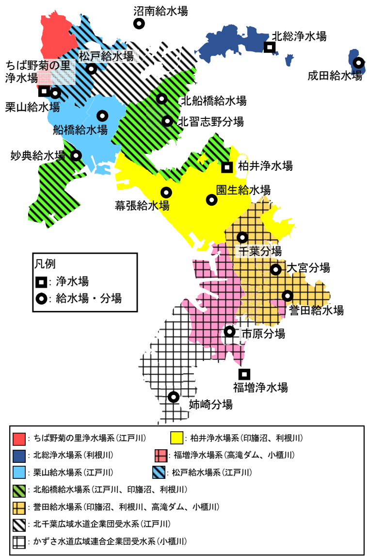
図6 配水系統図
