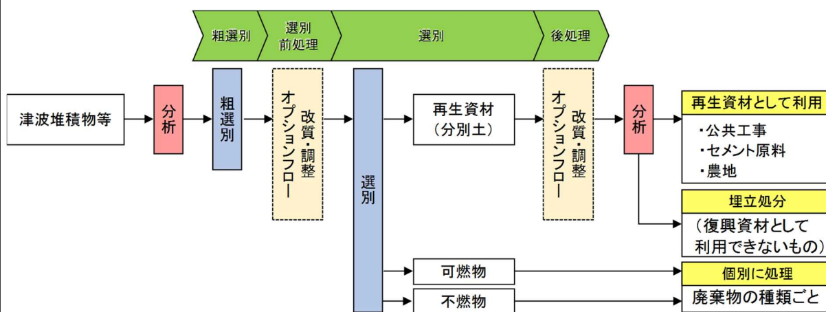
図表 2-25 津波堆積物処理フローの一般的な流れ
