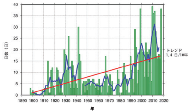
銚子地方気象台における真夏日日数の経年変化
