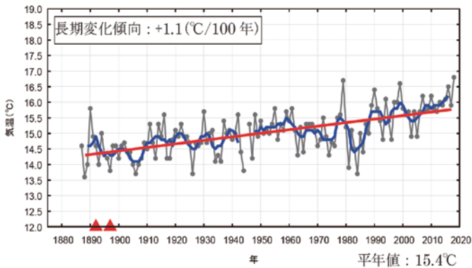
銚子地方気象台における年平均気温の経年変化
