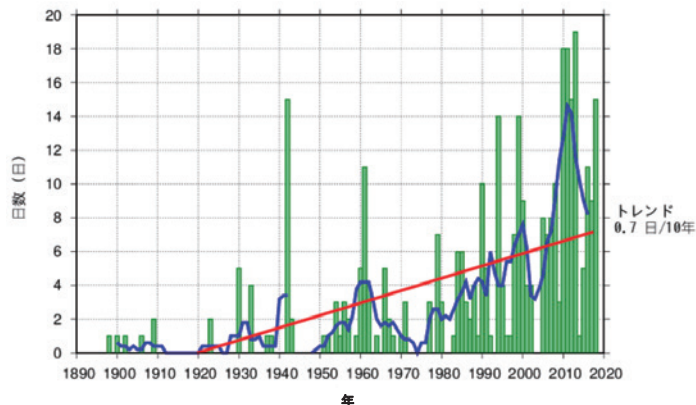
銚子地方気象台における熱帯夜日数の経年変化
