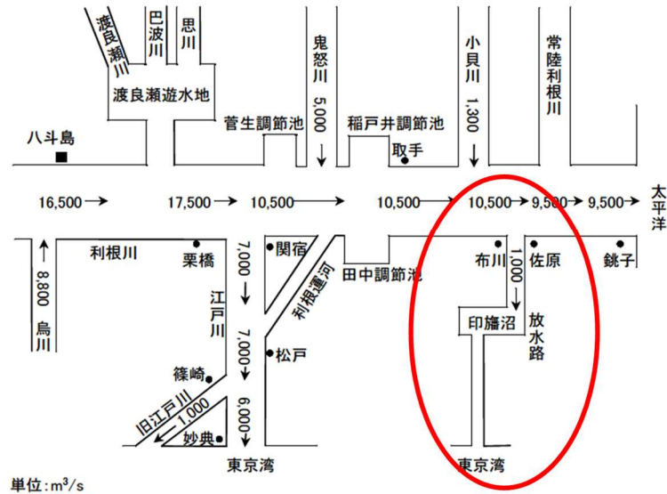
利根川計画高水流量図
