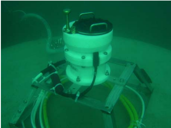
超音波式波高計
