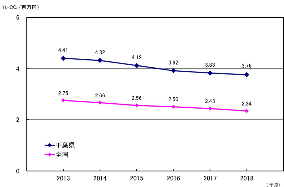
図 2-3 県民総生産百万円当たり温室効果ガス排出量の推移
