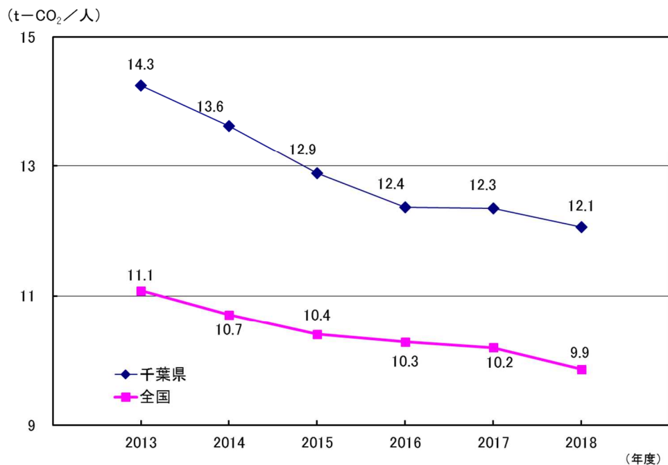
図 2-2 県民一人当たり温室効果ガス排出量の推移
