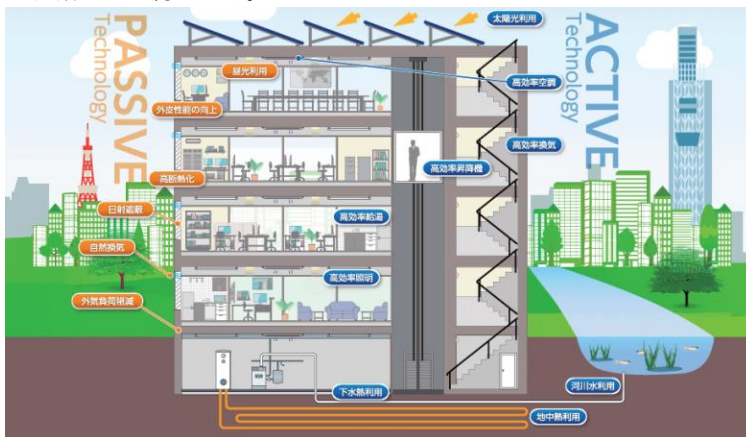
図：ZEB 出典：「ZEB PORTAL」(環境省)
